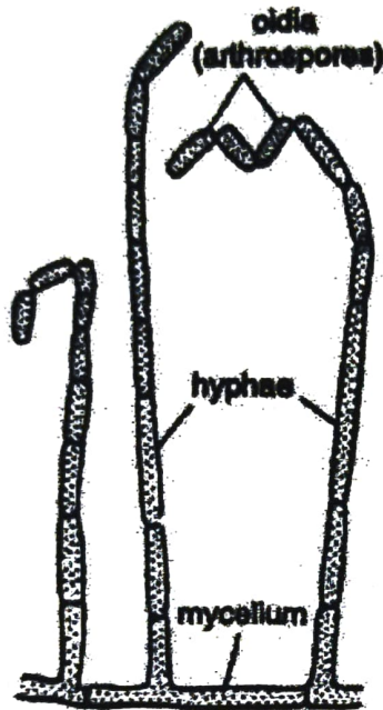
Fig. 2. Ascobolus : Arthrospores formation
