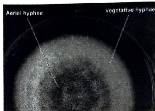
(b) A. niger on agar
